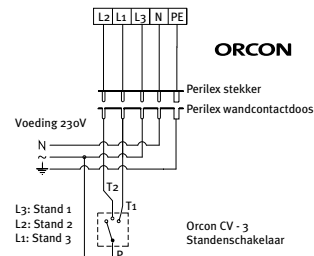
fig.6 Aansluitschema Compact-10P
