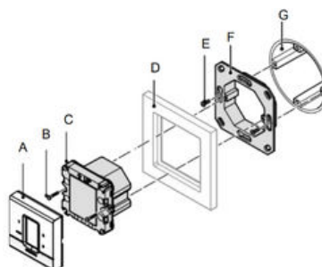
Figuur 1 Vocht Bedieningssensor Inbouw 15RF en toebehoren
