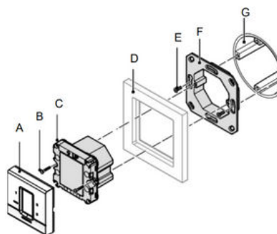
Figuur 1 Bewegingssensor Inbouw 15RF en toebehoren
