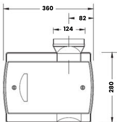
Vooraanzicht
