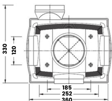
Achteraanzicht
